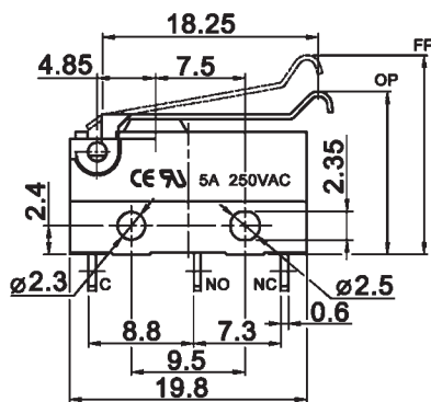
Actuator 04
