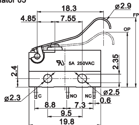
Actuator 05
